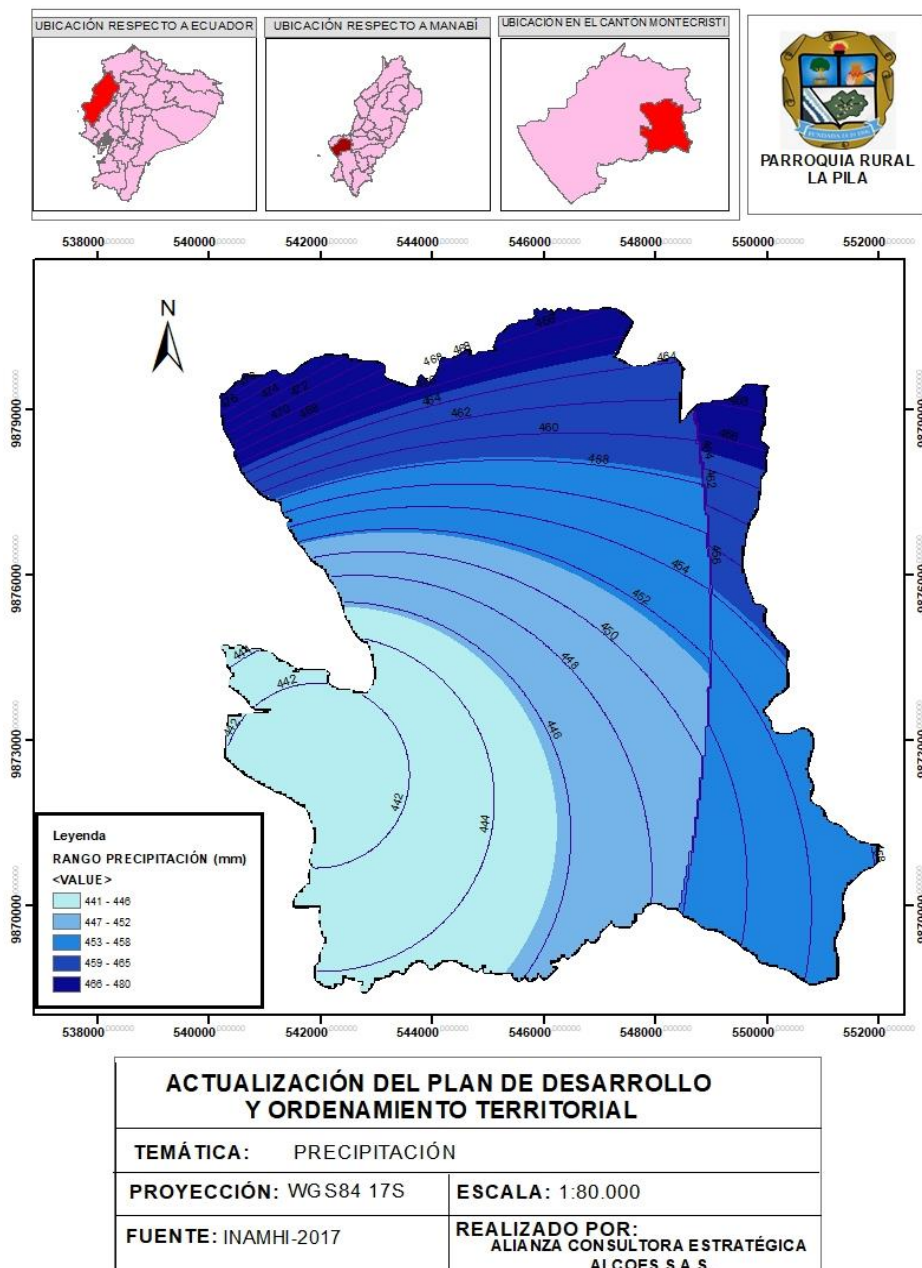
Mapa 12. Precipitación
