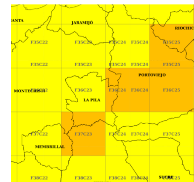
RCP 8.5 2016-2040 (ESCENARIO PESIMISTA)
